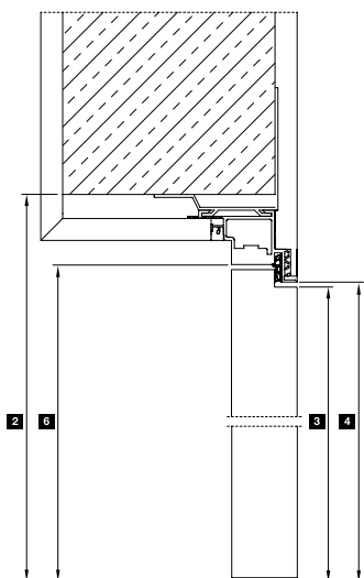
Vertikalschnitt mit reverse-öffnendem Türblatt
