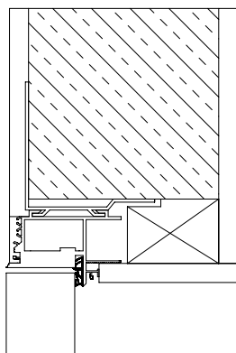
Horizontalschnitt mit stumpf einschlagender Tür
