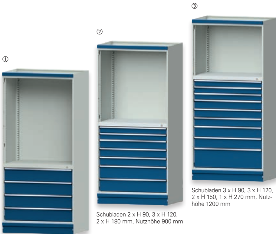
① Schubladen 4 x H 180 mm, Nutzhöhe 720 mm
