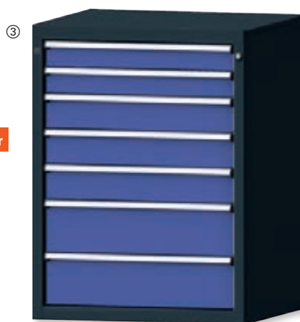
Breite 760 mm, 7 Schubladen 2 x 90, 3 x 120, 2 x 180 mm
